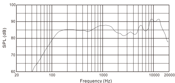
CMX6203 频率响应曲线
