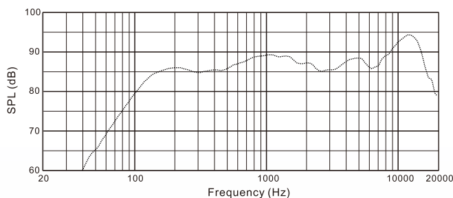
CMX6403 频率响应曲线
