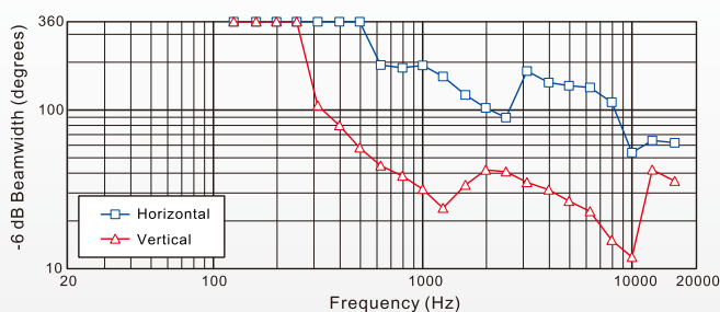
CMX6903 覆盖范围曲线
