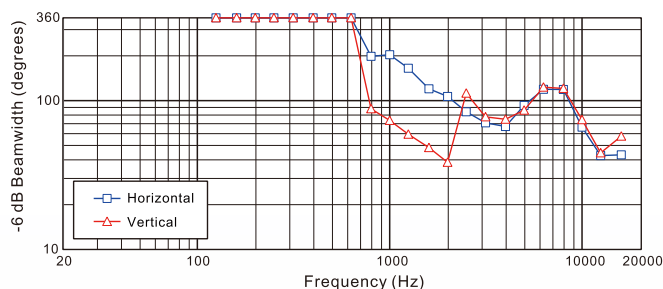
CMX6403 覆盖范围曲线
