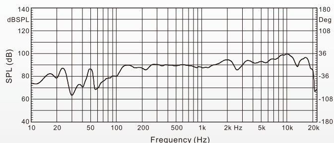
CMX6903 频率响应曲线
