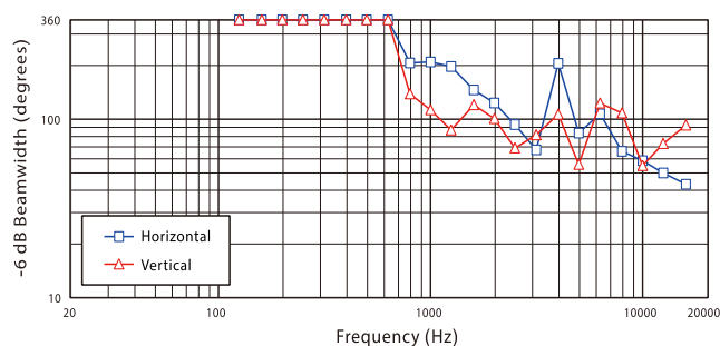
CMX6203 覆盖范围曲线
