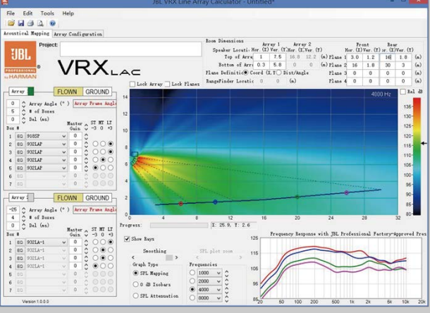
侧视图 (4 x VRX932LAP + 1 x VRX918SP) :
